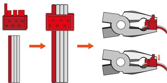
Figura 9 Crimpar conector para cable RS-485
