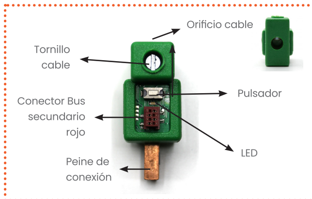
Figura 2 Descripción gráfica CcM1-C.
