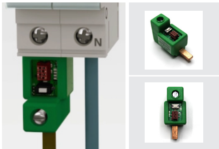
Figura 1 Aspecto del dispositivo CcM1-C.
