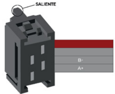
Figura 13: Conector RS-485
