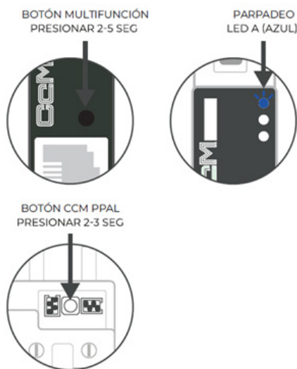
Figura 17: Proceso de asignación de ID Modbus
