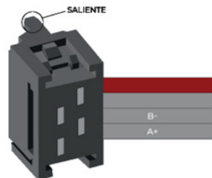
Figura 13: Conector RS-485
