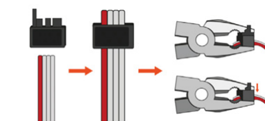
Figura 12: Crimpar conector para cable RS-485
