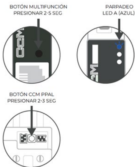
Figura 16: Proceso de asignación de ID Modbus
