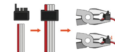
Figura 12: Crimpar conector para cable RS-485
