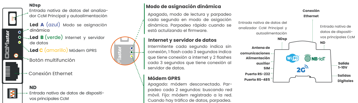
Figura 2: Descripción gráfica CcMaster
