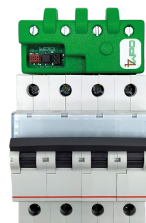
Figura 6: CcM4 instalado en magnetotérmico
