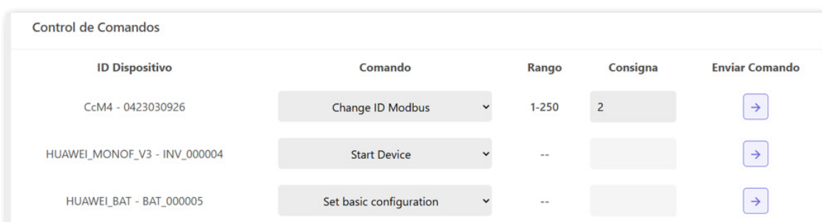
Figura 23: Web server – Automatización – Control Manual – Control de comandos
