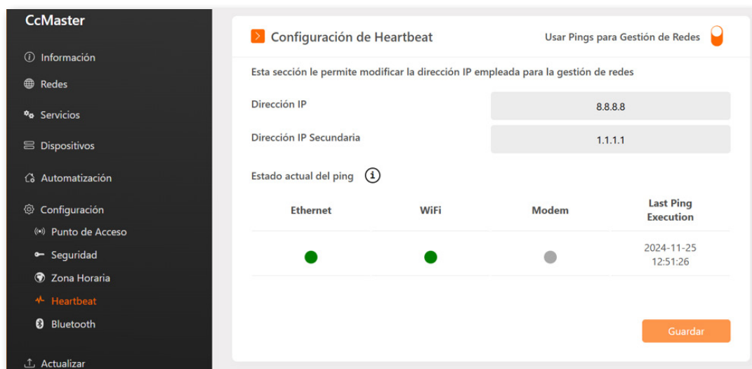
Figura 43: Web server – Configuración – Heartbeat
