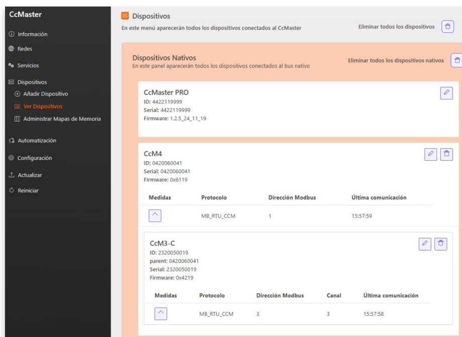
Figura 14: Web server – Dispositivos – Ver Dispositivos – Dispositivos Nativos
