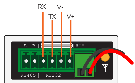
Figura 3 Pinout conector RS-232
