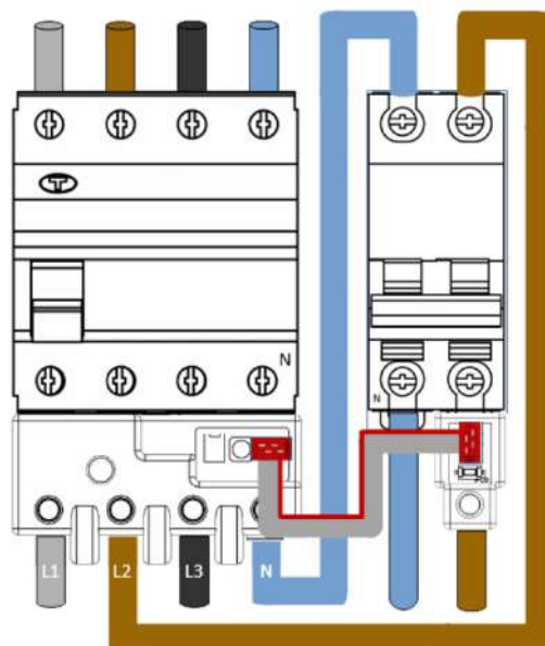
Figura 18 Conexión bus secundario
