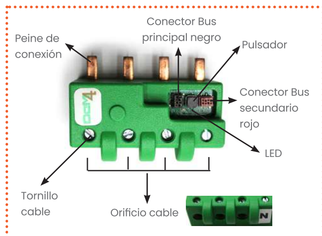
Figura 2 Descripción gráfica CcM4.
