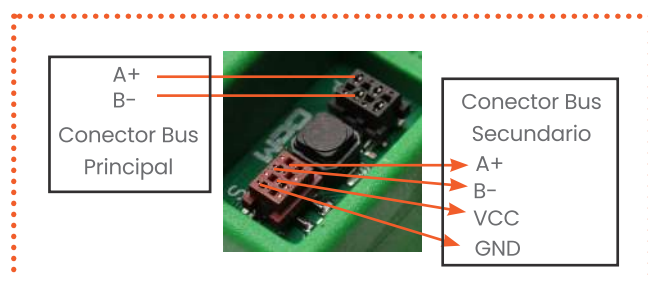
Figura 3 Detalle de los conectores CcM4.
