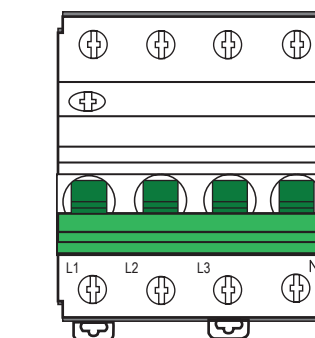
Figura 6 Interruptor magnetotérmico
