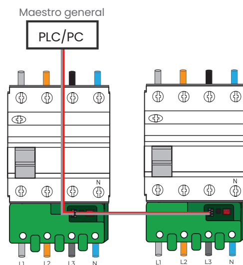
Figura 17 Conexión bus principal CcM4
