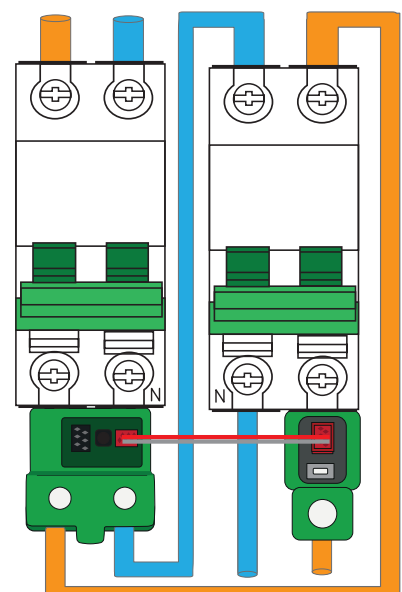
Figura 17 Conexión bus secundario
