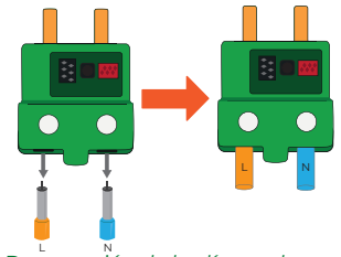
Figura 8 Desconexión de las líneas de corriente
