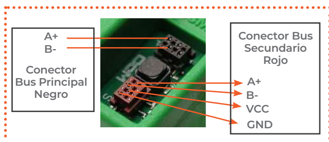
Figura 3 Detalle de los conectores CcM2 .
