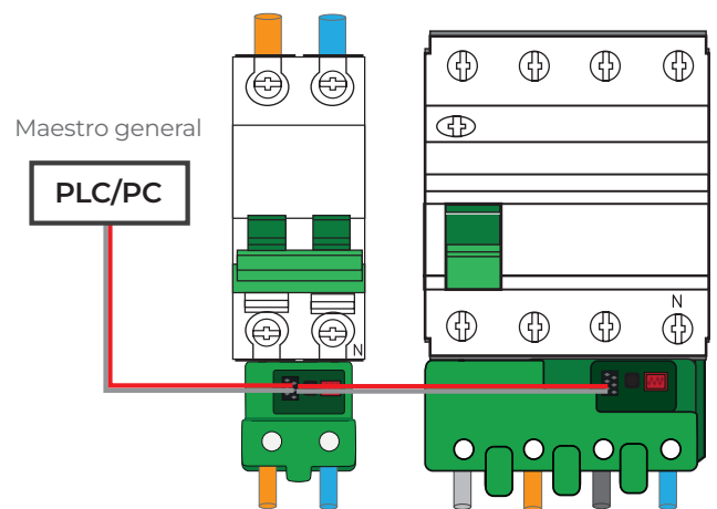
Figura 16 Conexión bus principal CcM2
