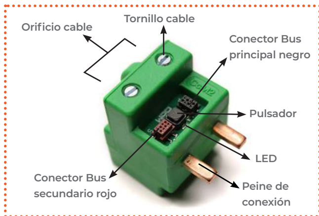
Figura 2 Descripción gráfica CcM2 .
