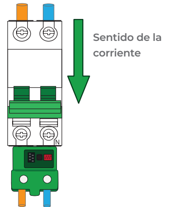
Figura 8 Desconexión de las líneas de corriente
