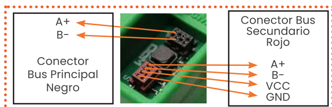
Figura 3 Detalle de los conectores CcM2
