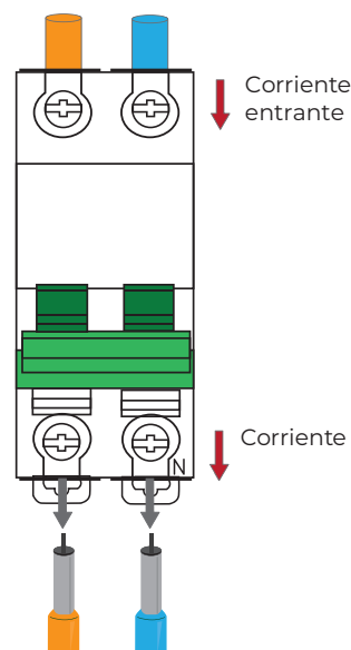
Figura 7 Desconexión de las líneas de corriente
