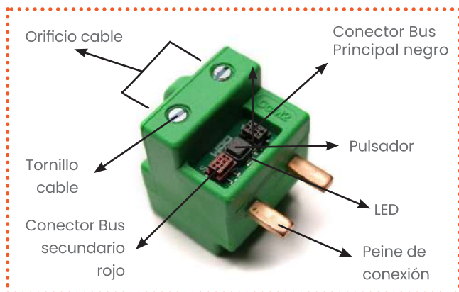
Figura 2 Descripción gráfica CcM2.
