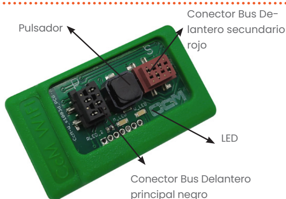
Figura 2 Descripción gráfica CcM-WIFI parte delantera.
