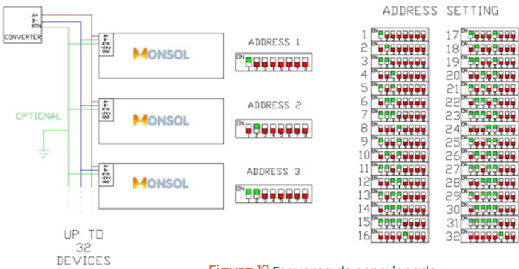
Figura 12 Esquema de conexionado
