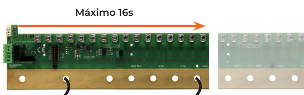
Figura 8 CcM-Shunt sin pletina de cobre o sobre embarado
