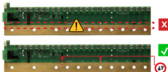
Figura 6 CcM-Shunt con remaches de nylon
