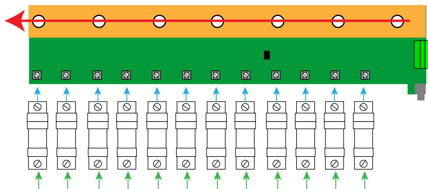
Figura 5 Diagrama de flujo de corriente
