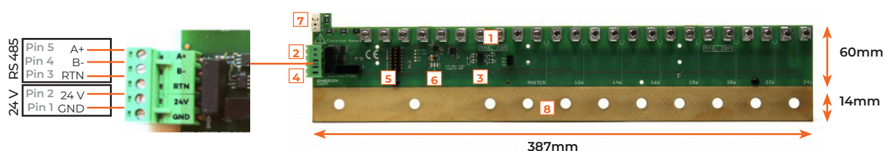
Figura 2 Componentes CcM-Shunt
