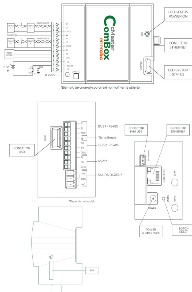
Figura 2: Descripción gráfica CcMaster Combox
