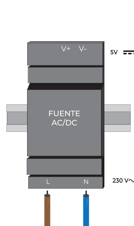
Figura 6: Conexión AC de la fuente de alimentación
