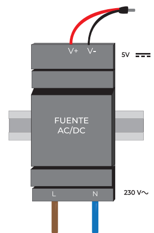
Figura 7: Conexión DC de la fuente de alimentación
