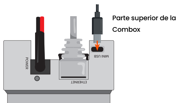
Figura 10: Conexión USB
