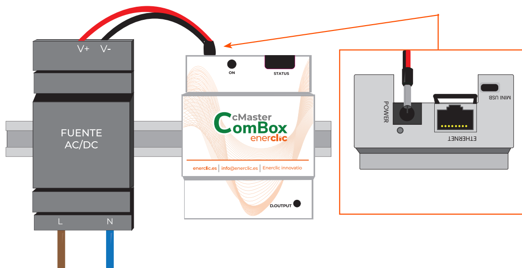
Figura 8: Conexión de latiguillo de alimentación a CcMaster Combox
