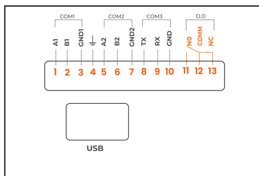
Figura 11: Conexiones puertos serie y salida digital
