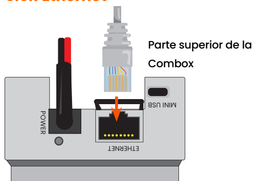
Figura 9: Conexión Ethernet
