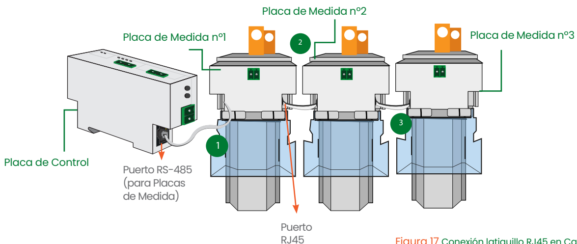
Figura 17 Conexión latiguillo RJ45 en Captador – Vista 3D
