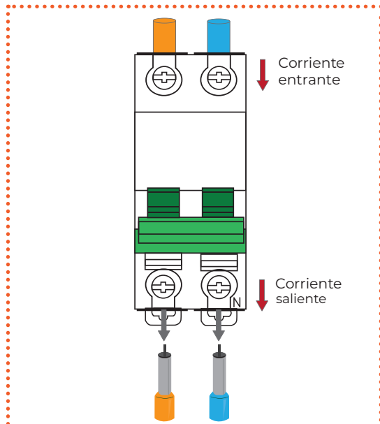
Figura 3 Desconexión de las líneas de corriente
